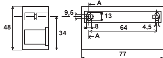
Transmitter 1007 Simple door version
