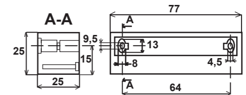
Sender 1007 Einzeln Tür Version
