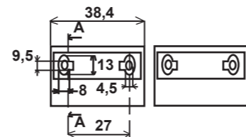
Transmitter 1007D Double hinge door version
